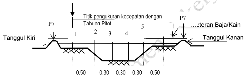
Contoh sketsa situasi sungai
