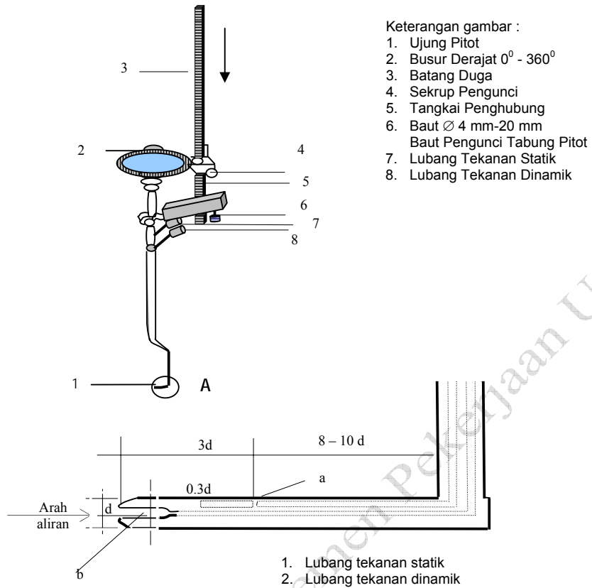
DETAIL A. UJUNG TABUNG PITOT
