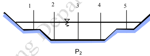
Gambar B.2 Penampang melintang sungai
