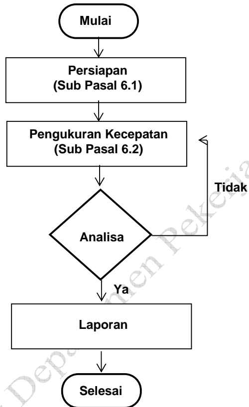
Gambar A.1 Bagan alir tata cara pengukuran kecepatan aliran pada uji model hidraulik fisik dengan tabung pitot
